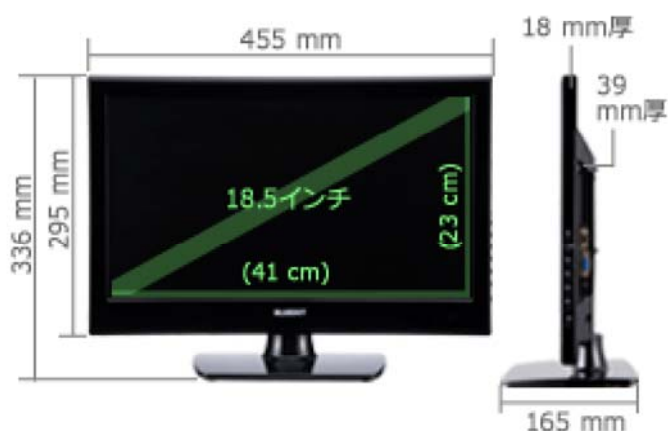
本体寸法
